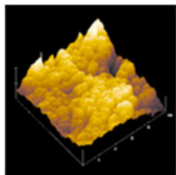
Mikrostruktur Lotusan
