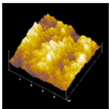
Mikrostruktur Lotusblatt
